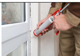
Luftdichter Abschluss innen
